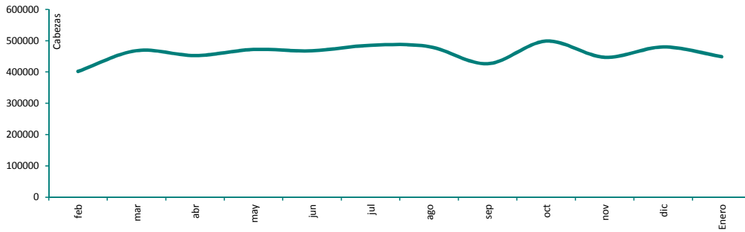
Gráfico 14: CAPONES FAENADOS
